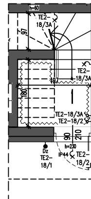
RZUT PARTERU
