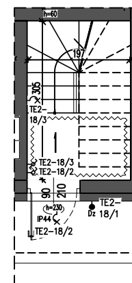
RZUT PARTERU
