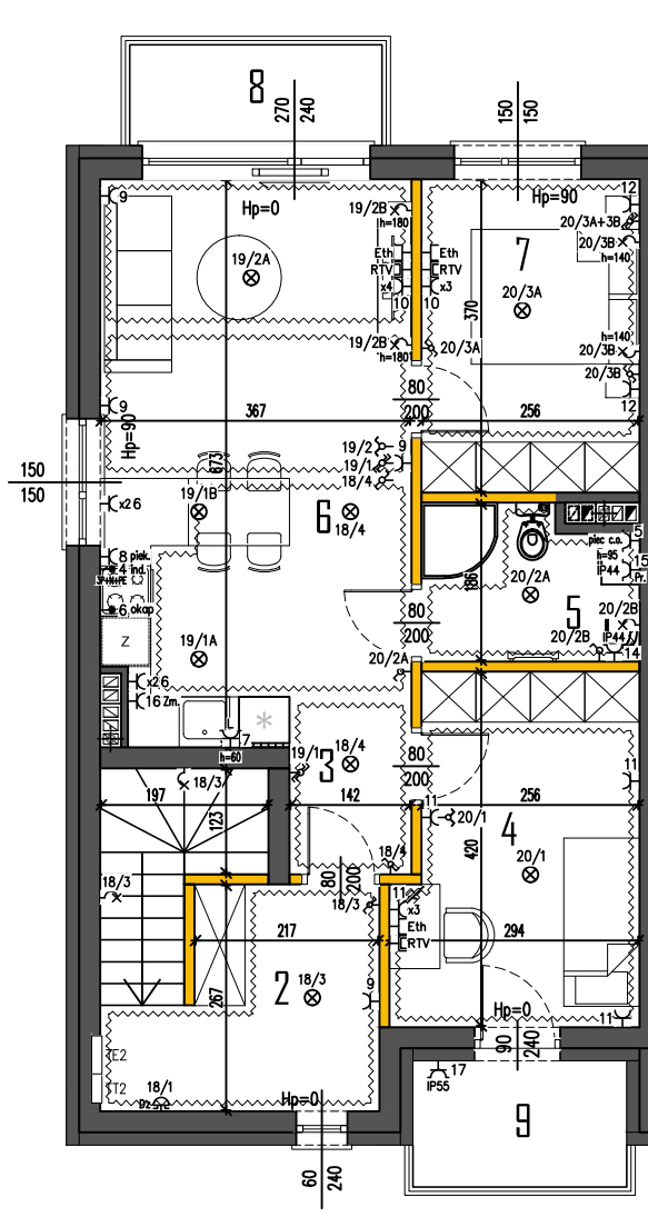
RZUT I PIĘTRA
