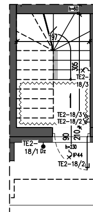
RZUT PARTERU
