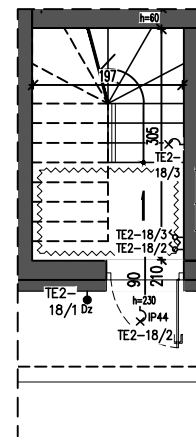
RZUT PARTERU
