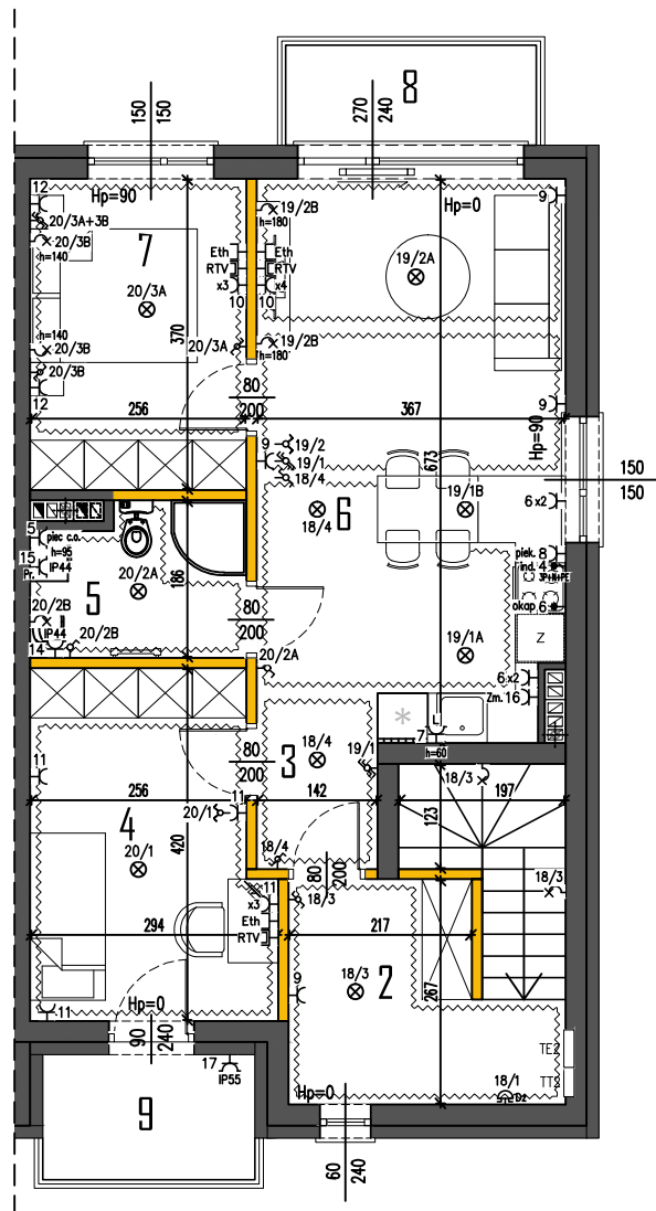
RZUT I PIĘTRA
