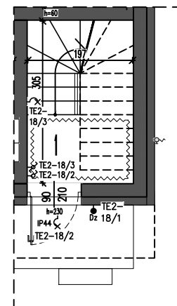
RZUT PARTERU
