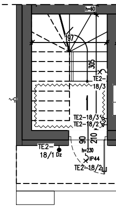
RZUT PARTERU
