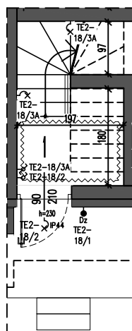
RZUT PARTERU
