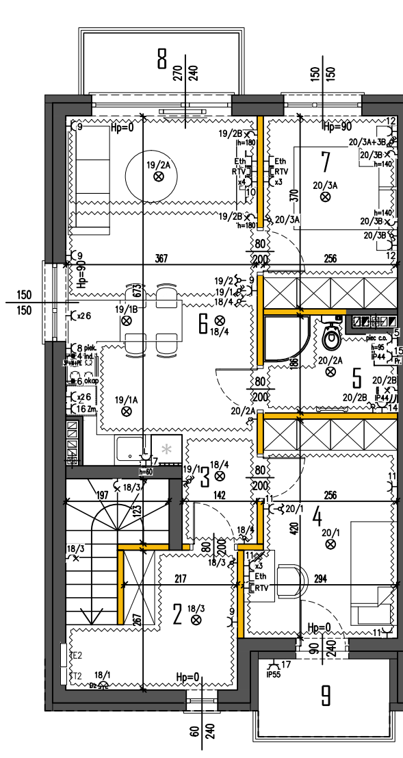
RZUT PIĘTRA
