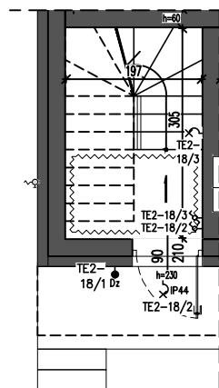
RZUT PARTERU
