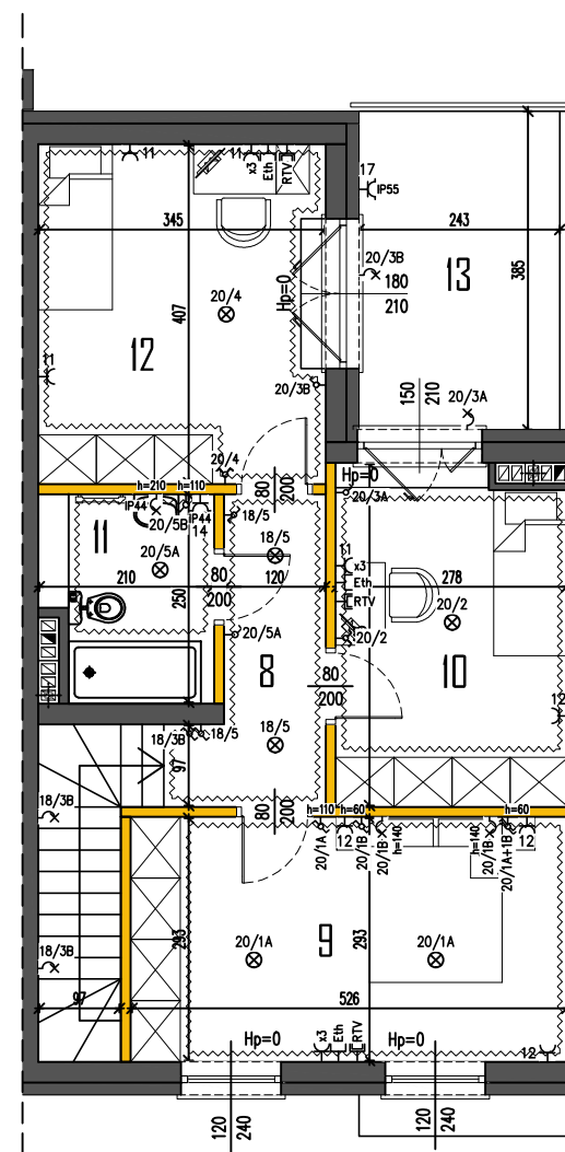
RZUT II PIĘTRA
