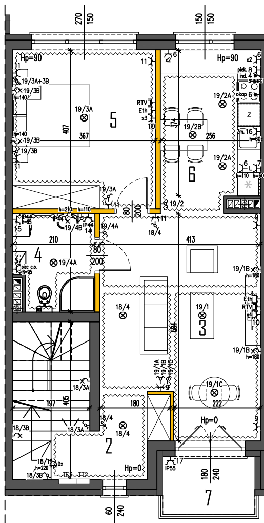
RZUT PIĘTRA
