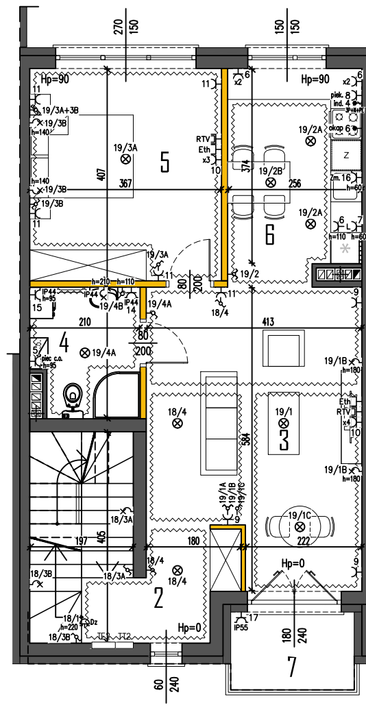
RZUT PIĘTRA
