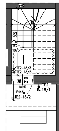
RZUT PARTERU
