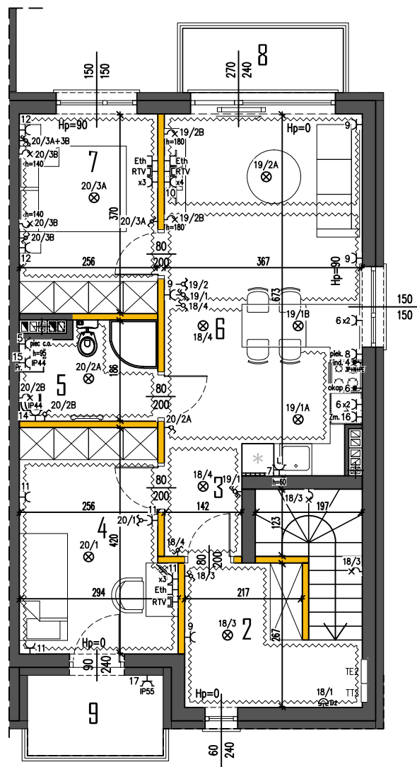
RZUT PIĘTRA
