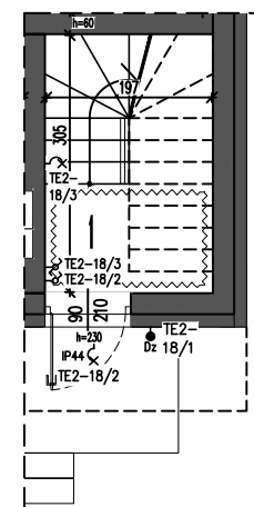
RZUT PARTERU
