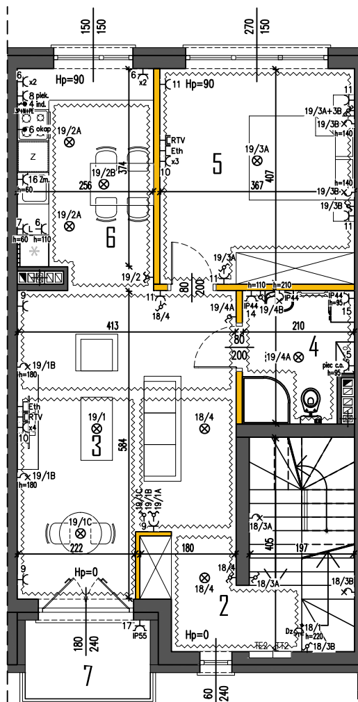
RZUT PIĘTRA
