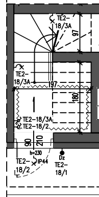
RZUT PARTERU
