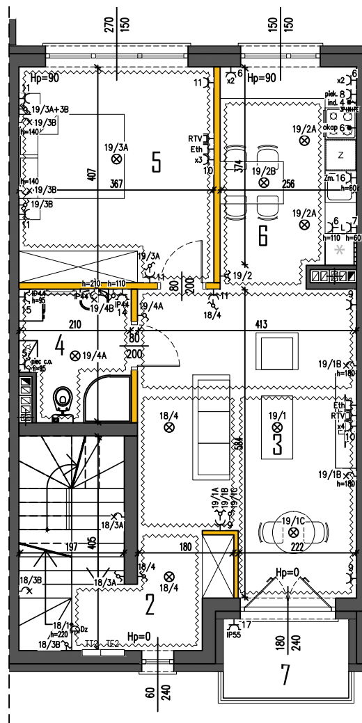
RZUT PIĘTRA
