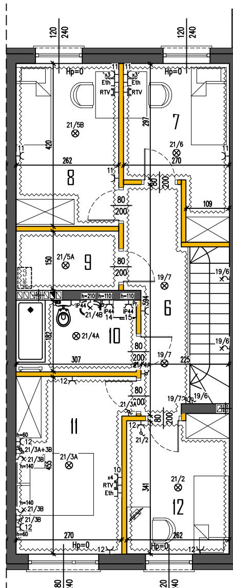
RZUT PIĘTRA
