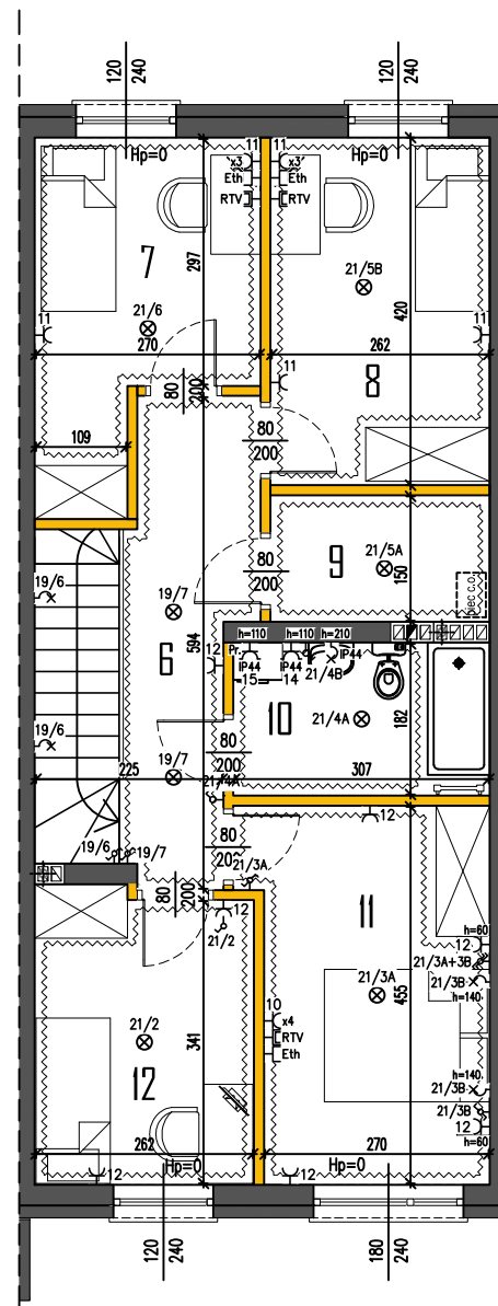
RZUT PIĘTRA
