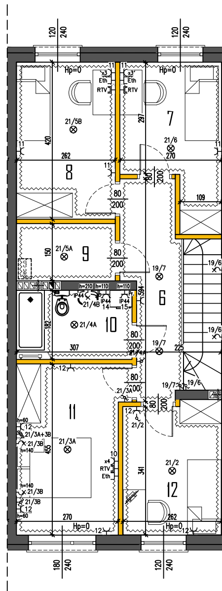
RZUT PIĘTRA
