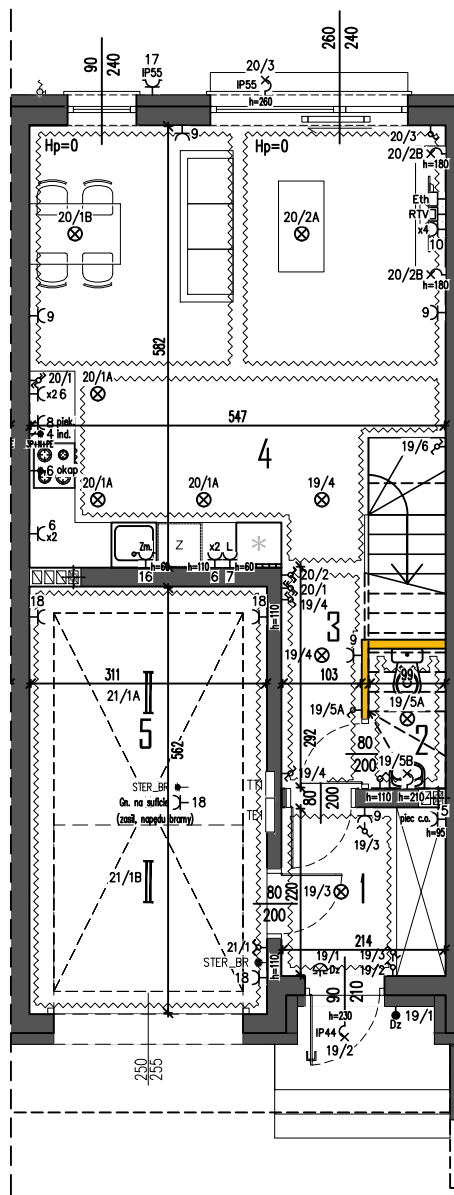
RZUT PARTERU
