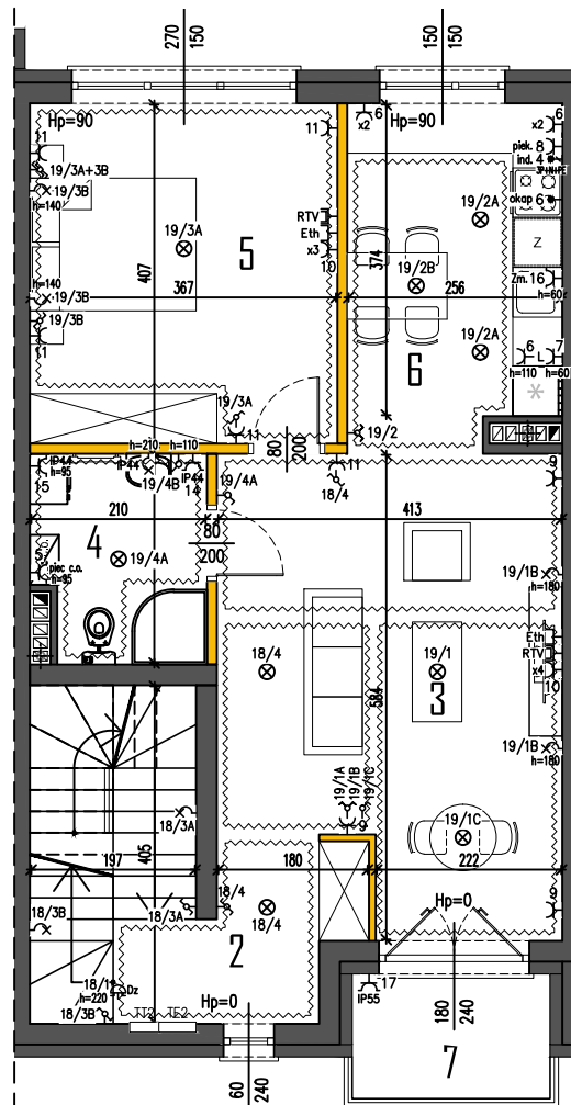
RZUT PIĘTRA
